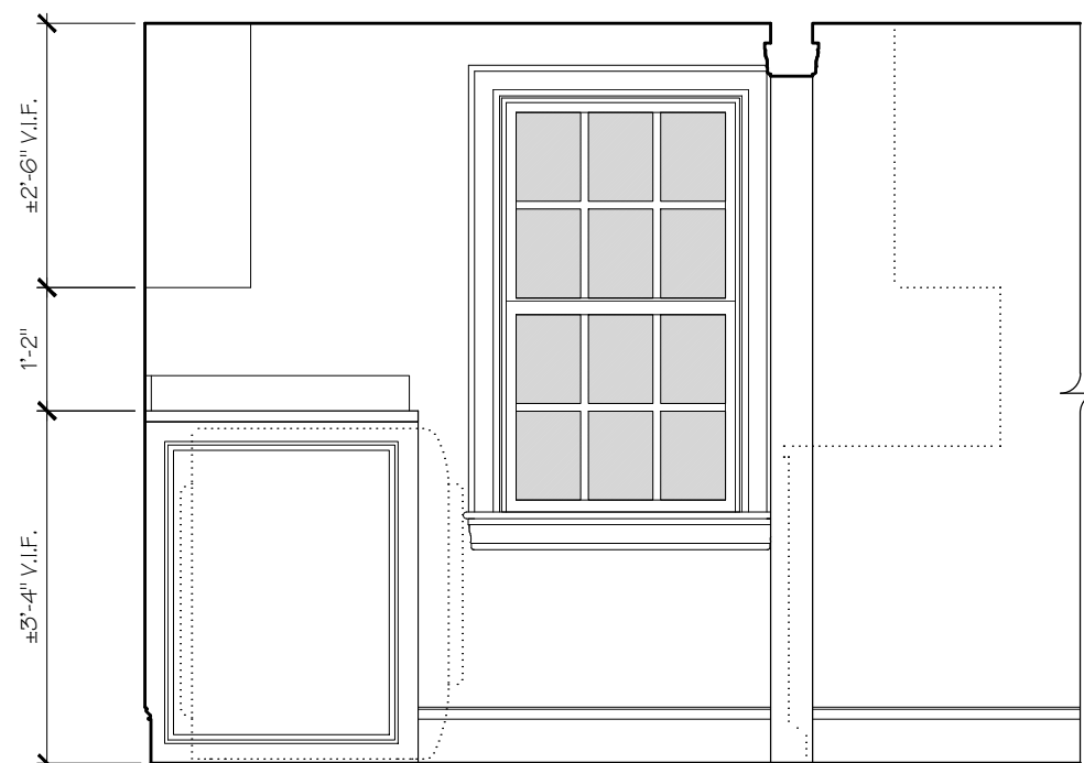
2A LAUNDRY A401 SCALE: 1/2" = 1'-0"
