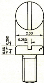
(d) Pan head
